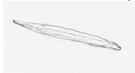
Oumuamua
